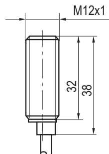
Габаритный чертеж
