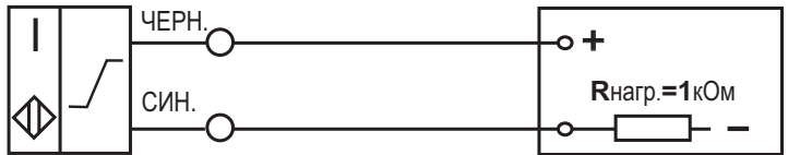
Схема подключения к оборудованию
